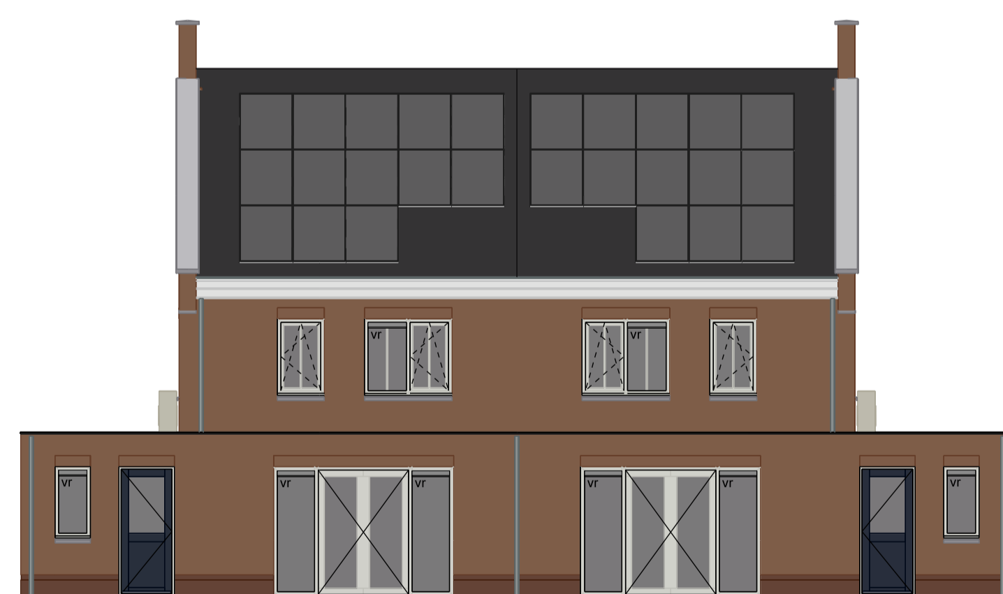
Achtergevel
