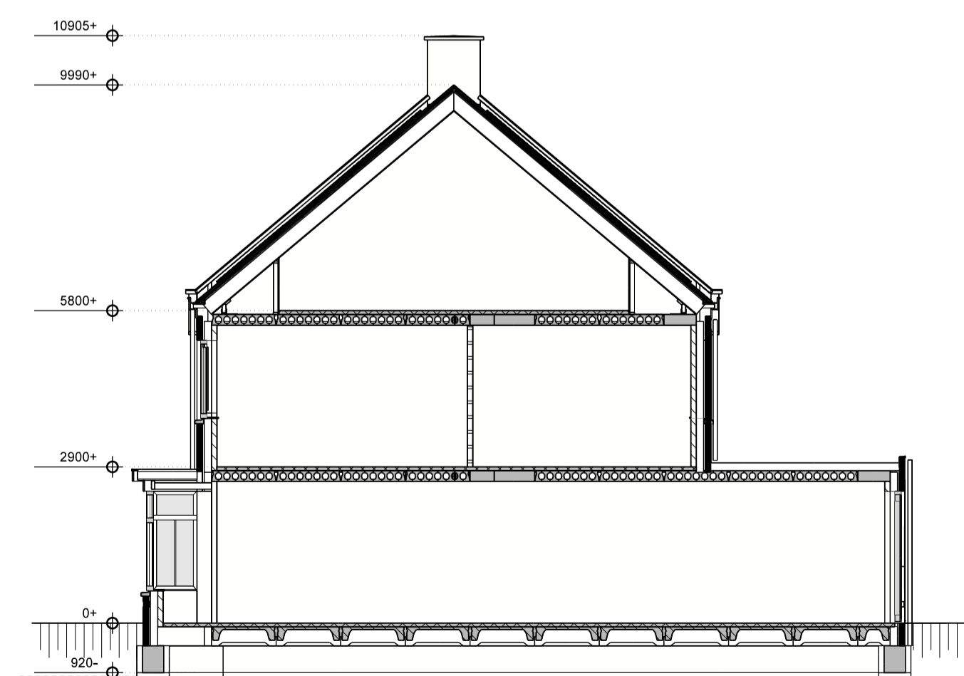
Doorsnede
